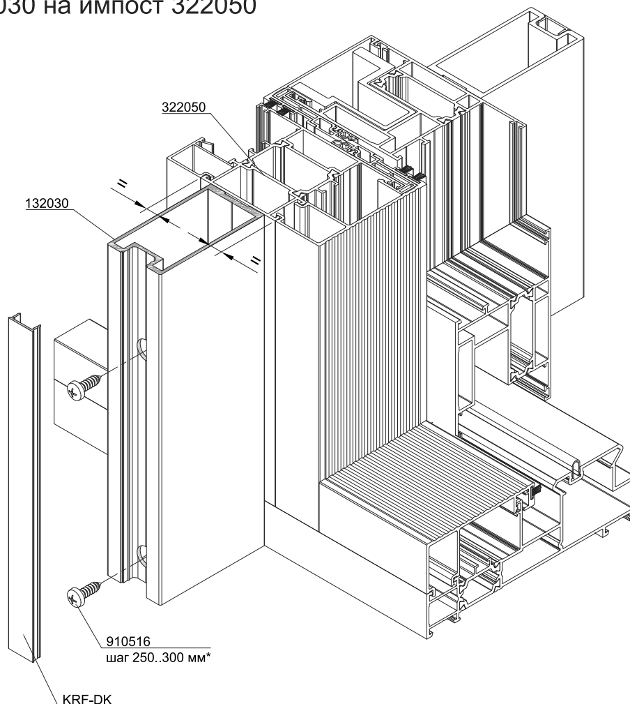
Обработка профиля усилителя 132030
