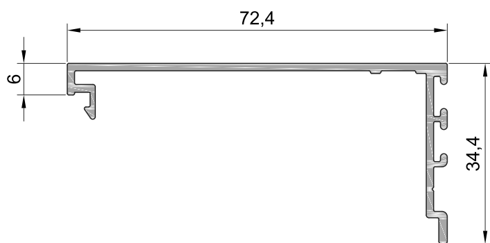
Профиль крышки створки
