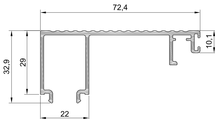
Профиль крышки рамы
