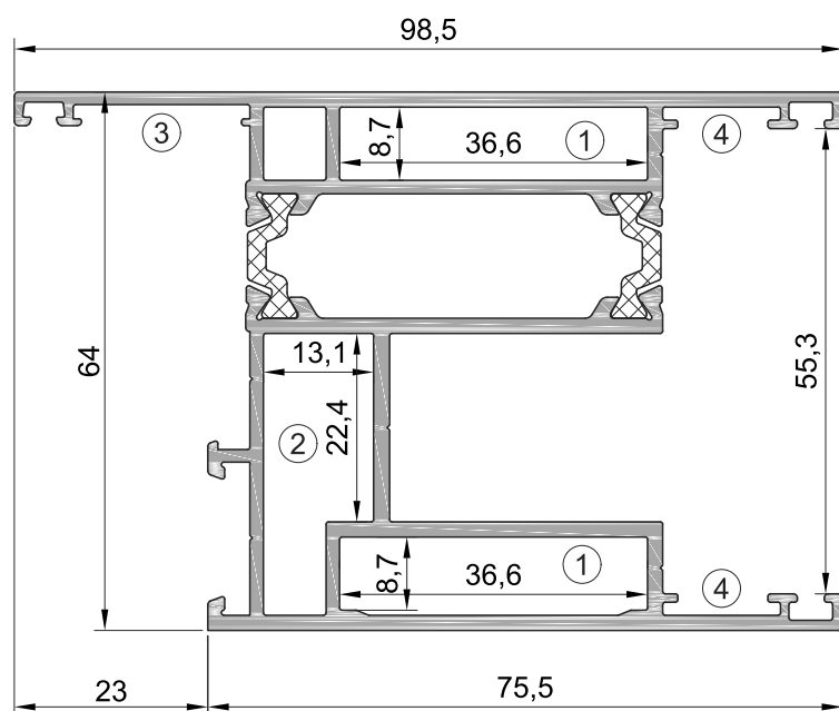
Створочный профиль 0,113
