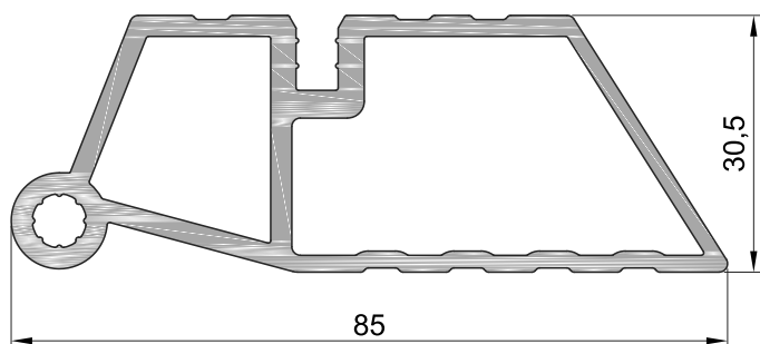
Профиль углового шарнирного соединителя 30,5 мм
