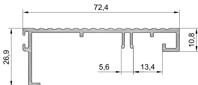
Профиль внутреннего порога
