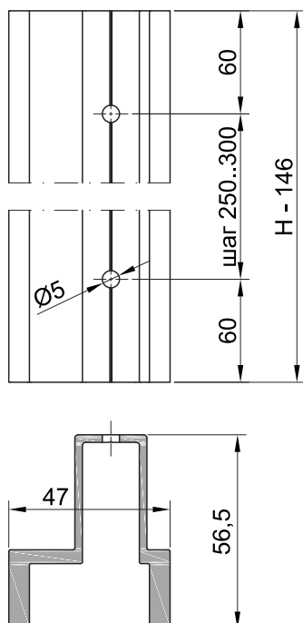
Обработка профиля усилителя 132020
