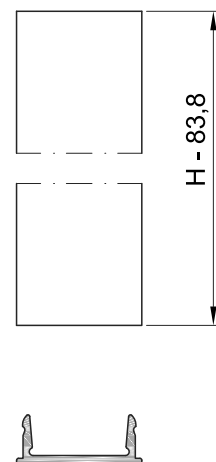
Обработка профиля декоративной крышки KRF-DK
