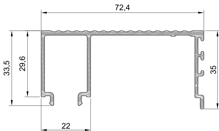
Профиль крышки импоста
