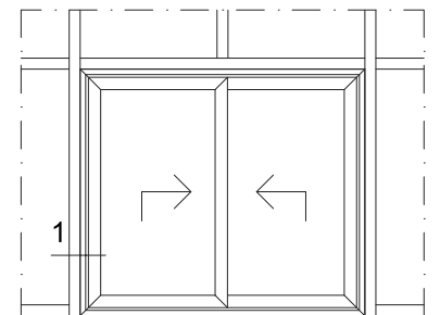
Подъемно-сдвижная конструкция встроенная в фасад
