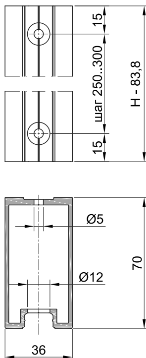
Обработка профиля усилителя 132030
