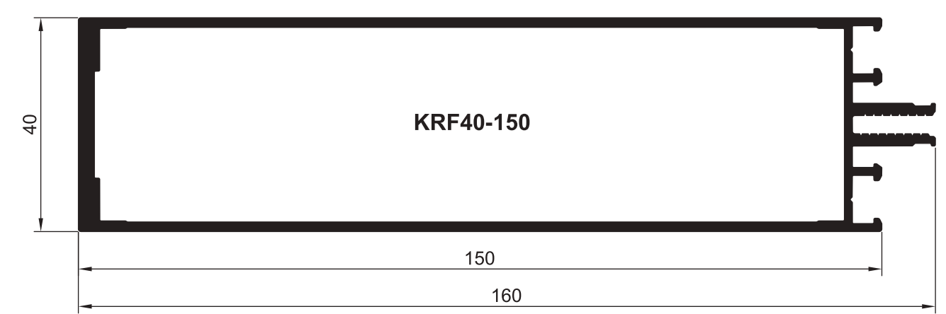
ПРОФИЛИ СТОЕК / РИГЕЛЕЙ
