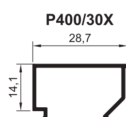
ПРОФИЛИ ШТАПИКОВ
