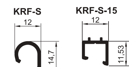
ПРОФИЛЬ ДИСТАНЦИОНЕРА
