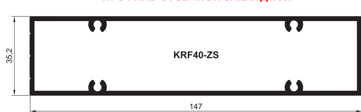
ПРОФИЛЬ РИГЕЛЬНОЙ ЗАКЛАДНОЙ
