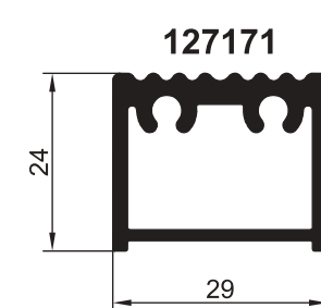
ПРОФИЛЬ УСИЛИТЕЛЯ
