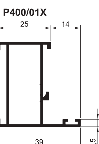
ПРОФИЛИ ОКОННЫЕ РАМНЫЕ
