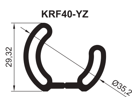
ПРОФИЛЬ РИГЕЛЬНОЙ ЗАКЛАДНОЙ
