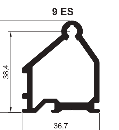
ПРОФИЛЬ ЗАКЛАДНОЙ
