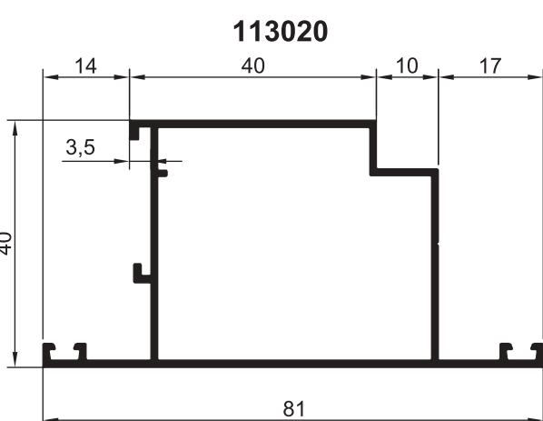
ПРОФИЛИ ДВЕРНЫЕ СТВОРОЧНЫЕ
