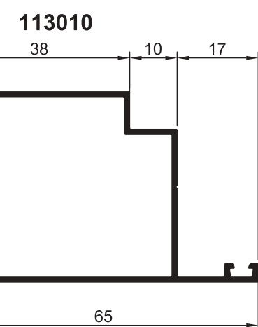
ПРОФИЛЬ ДВЕРНОЙ РАМНОЙ
