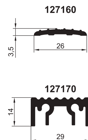
ПРОФИЛЬ ПОРОГА
