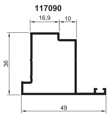
ПРОФИЛЬ ДВЕРНОЙ ШТУЛЬПОВЫЙ
