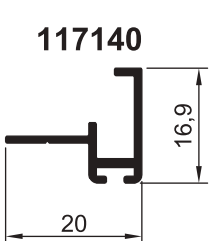
ПРОФИЛИ ШТАПИКОВ
