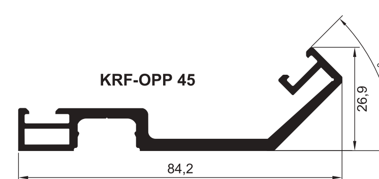
ПРОФИЛИ ДЕКОРАТИВНЫХ КРЫШЕК
