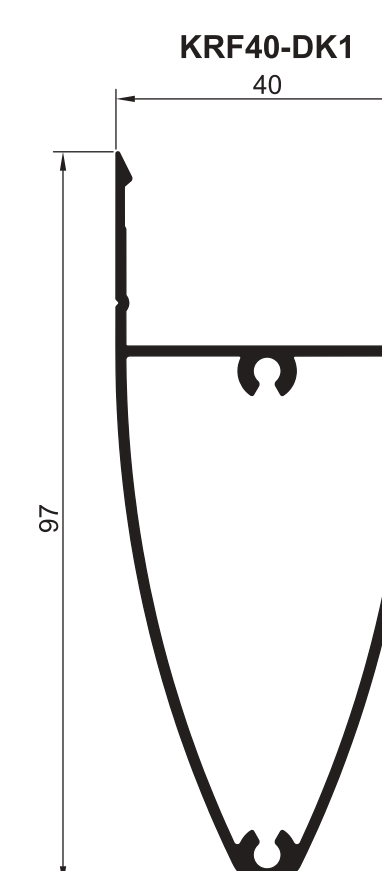
ПРОФИЛИ ДЕКОРАТИВНЫХ КРЫШЕК
