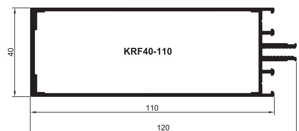
ПРОФИЛЬ РИГЕЛЬНОЙ ЗАКЛАДНОЙ
