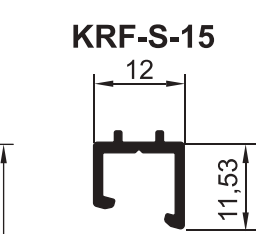
ПРОФИЛЬ ДИСТАНЦИОНЕРА
