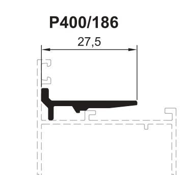
ПРОФИЛЬ ПОДКЛАДКИ ПОД СТЕКЛОПАКЕТ
