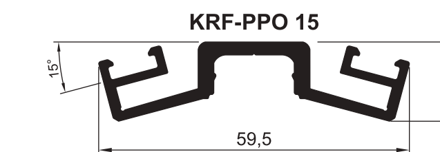
ПРОФИЛИ ПРИЖИМНЫХ ПЛАНК
