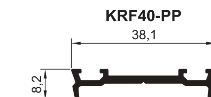
ПРОФИЛИ ПРИЖИМНЫХ ПЛАНК
