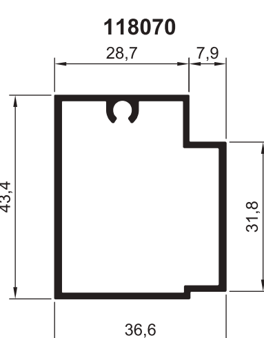
ПРОФИЛЬ УСИЛИТЕЛЯ
