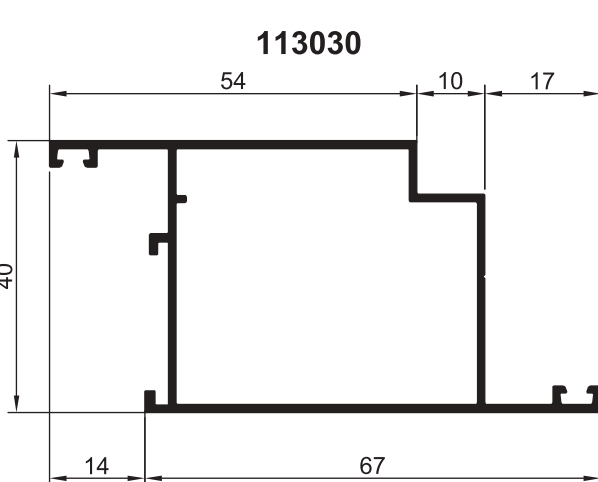
ПРОФИЛИ ОКОННЫЕ РАМНЫЕ
