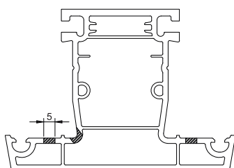
13.7 Вентиляционные отверстия, импост.
