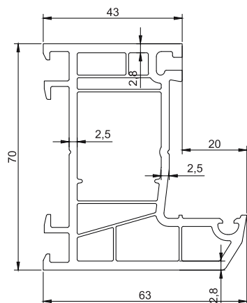
3.1.5 Профиль рамы арт. 7501 A
