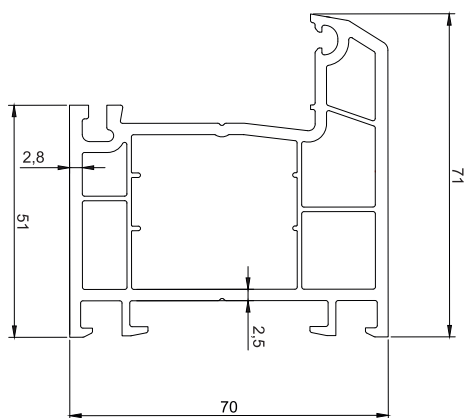
5.2.1 Профиль рамы дверной арт. 7004
