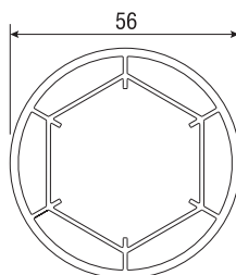
2.1.15 Профиль трубы для эркерных окон арт. 5814
