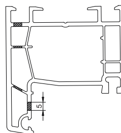
13.4 Вентиляционные отверстия, рама по бокам.
