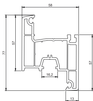
2.1.14 Профиль створки арт. 5802-13
