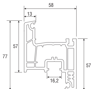
2.1.2 Профиль створки арт. 5802 A
