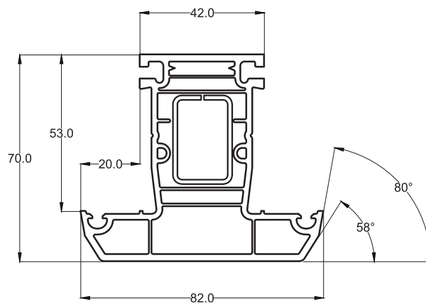
3.1.8 Профиль импоста арт. 7503
