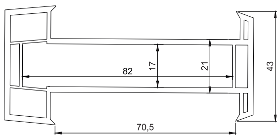
3.1.18 Статический усилитель арт. 7019
