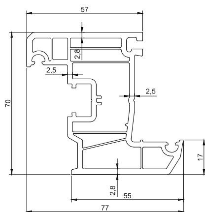
3.1.7 Профиль створки арт. 7502 А
