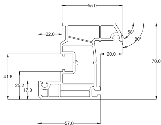
3.1.6 Профиль створки арт. 7502
