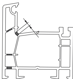
13.1 Вентиляционные отверстия, рама внизу. Вариант 1
