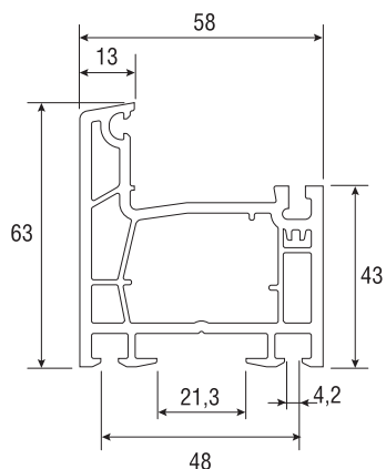
2.1.1 Профиль рамы арт. 5801 A
