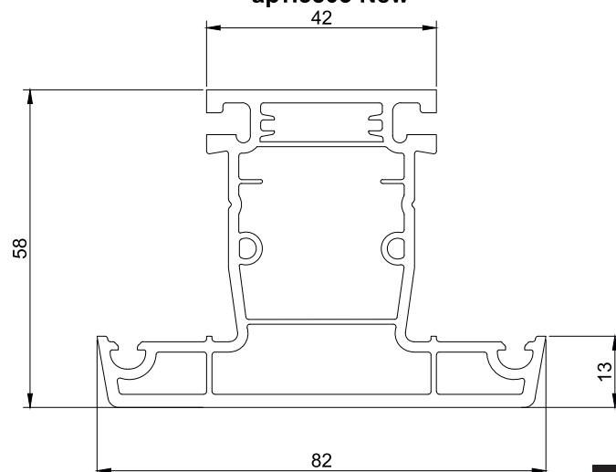
2.1.22 Профиль импоста арт.5803 New
