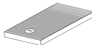
3.1.22 Опорная прокладка под стеклопакет 40 мм, 1 мм, 2 мм, 3 мм, 4 мм, 5 мм, серии 7000 арт. K721, K722, K723, K724, K725
