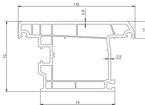
5.2.2 Профиль створки дверной наружного открывания арт. 7005
