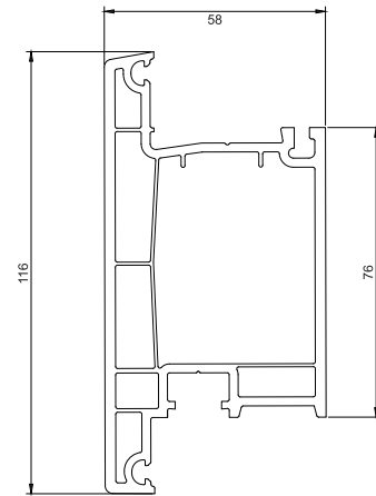
4.2.2 Профиль створки дверной наружного открывания арт. 5805
