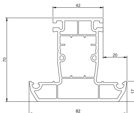
5.2.3 Профиль импоста арт. 7303
