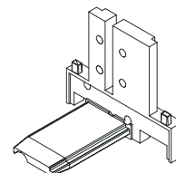
5.2.5 Соединитель дверной рамы и порога арт. K70
