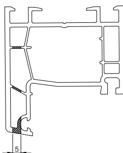
13.3 Вентиляционные отверстия, рама вверху.
