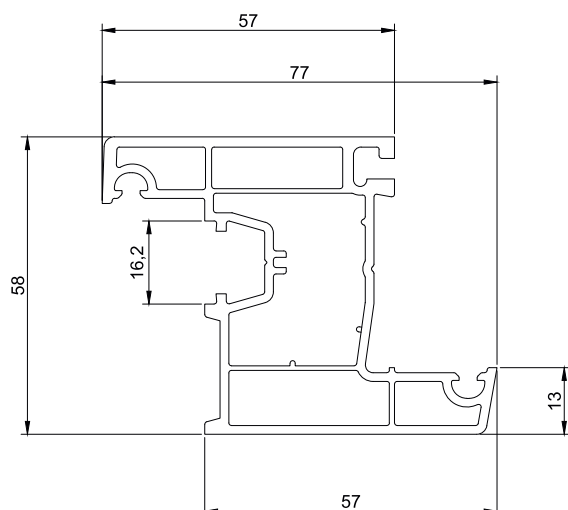
2.1.20 Профиль створки арт.5802 New
