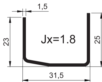
7.8 Армирующий профиль для арт. 5814 арт. K640
