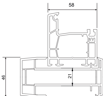
2.1.18 Статический усилитель арт.5819
