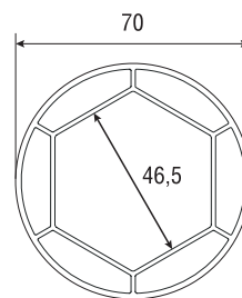
3.1.15 Труба ПВХ для эркерных окон арт. 7014
