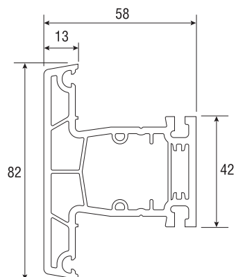
2.1.3 Профиль импоста арт. 5803 A
