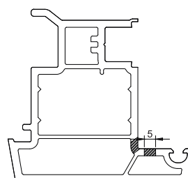
13.8 Вентиляционные отверстия, штульп.
