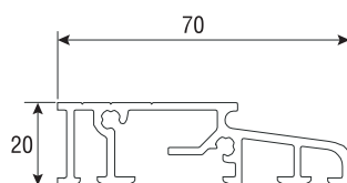
5.2.4 Порог алюминиевый арт. 7011
