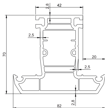
3.1.9 Профиль импоста арт. 7503 А
