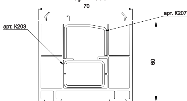
3.1.19 Профиль расширительный 60 мм арт. 7060
