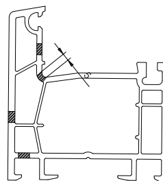
13.2 Вентиляционные отверстия, рама внизу. Вариант 2
