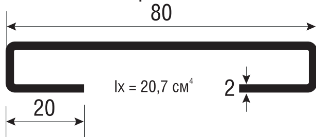
7.7. Армирующий профиль для арт. 5871 арт. r 208
