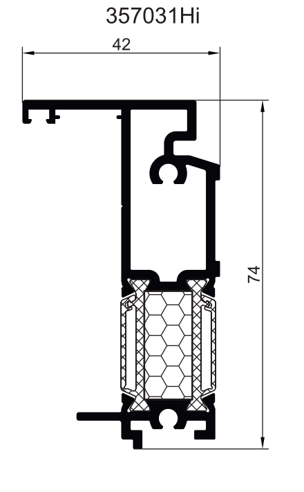
ПРОФИЛЬ ДВЕРНОЙ ШТУЛЬПОВЫЙ - ОТКРЫВАНИЕ НАРУЖУ
