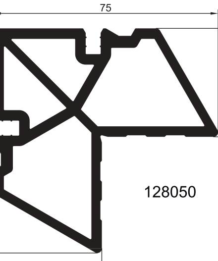
ПРОФИЛЬ ОПОРЫ
