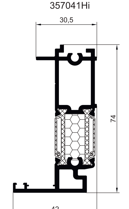
ПРОФИЛЬ ДВЕРНОЙ ШТУЛЬПОВЫЙ - ОТКРЫВАНИЕ ВНУТРЬ
