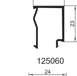
ПРОФИЛЬ РАМНОЙ АНТИМОСКИТНОЙ СЕТКИ
