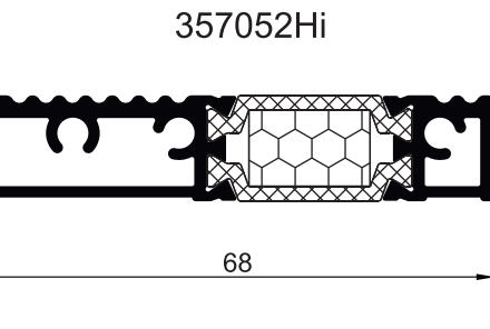
ПРОФИЛИ ПОРОГА
