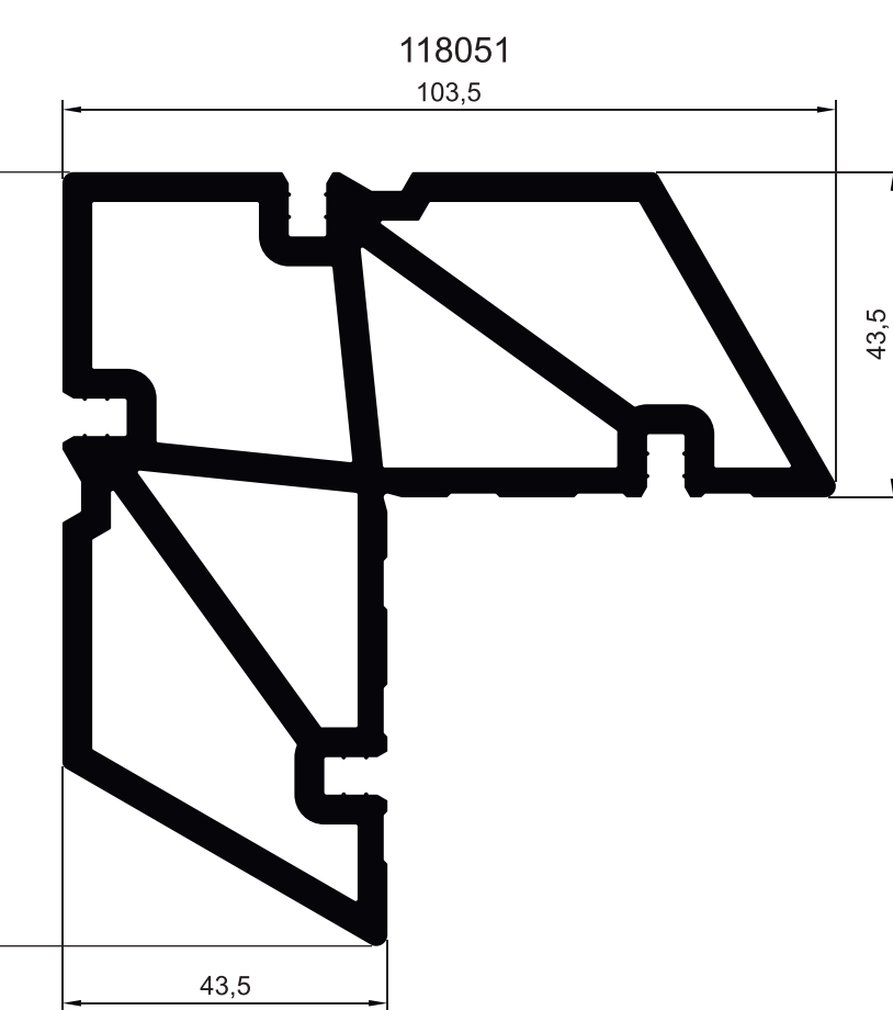
ПРОФИЛЬ УГЛОВОГО СОЕДИНЕНИЯ
