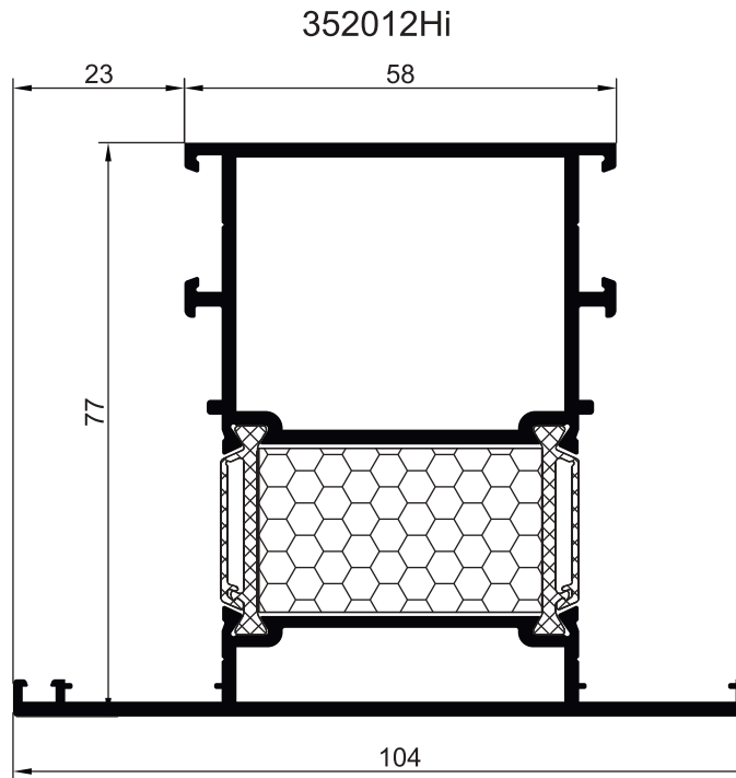
ПРОФИЛЬ ДВЕРНОЙ ИМПОСТНЫЙ
