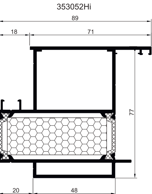
ДВЕРНОЙ РАМНОЙ ПРОФИЛЬ В ФАСАД - ОТКРЫВАНИЕ ВНУТРЬ
