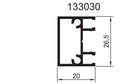
ПРОФИЛЬ КРЫШКИ АНТИМОСКИТНОЙ СЕТКИ
