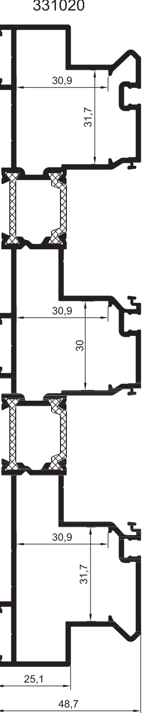
ПРОФИЛЬ РАМНОЙ МОНОРЕЛЬСОВЫЙ
