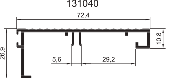
ПРОФИЛЬ ВНУТРЕННЕГО ПОРОГА
