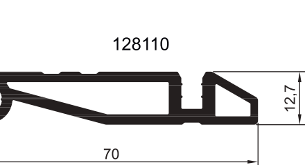
ПРОФИЛЬ УГЛОВОГО ШАРНИРНОГО СОЕДИНИТЕЛЯ
