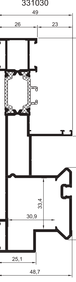
ПРОФИЛЬ РАМНОЙ МОНОРЕЛЬСОВЫЙ
