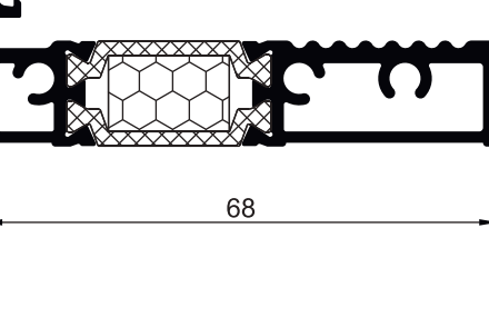
ПРОФИЛЬ ДВЕРНОЙ ШТУЛЬПОВЫЙ - ОТКРЫВАНИЕ ВНУТРЬ
