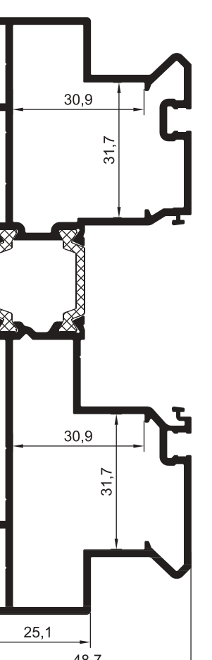
ПРОФИЛЬ РАМНОЙ ТРЕХРЕЛЬСОВЫЙ
