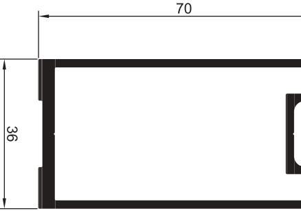
ПРОФИЛЬ РАМНОЙ АНТИМОСКИТНОЙ СЕТКИ
