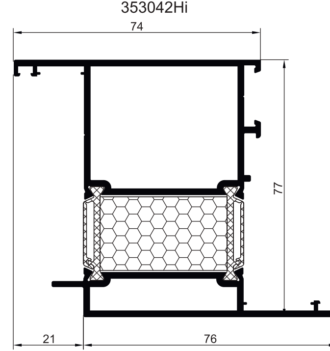
ПРОФИЛЬ ДВЕРНОЙ СТОВРОЧНЫЙ Z - ОБРАЗНЫЙ ПРОФИЛЬ
