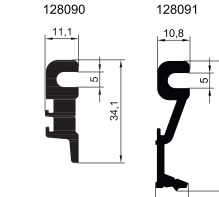
ПРОФИЛИ Т-ОБРАЗНОГО СОЕДИНИТЕЛЯ
