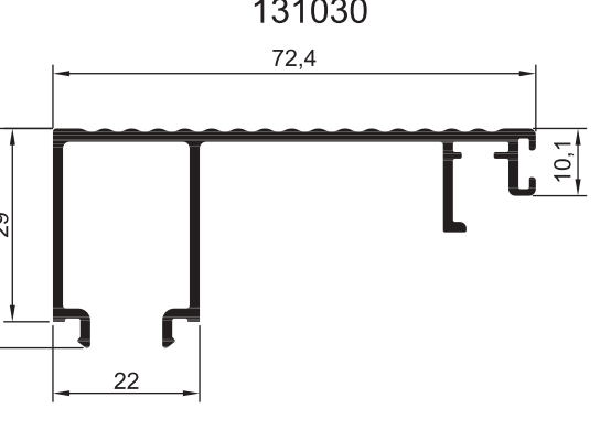
ПРОФИЛЬ НАРУЖНОГО ПОРОГА
