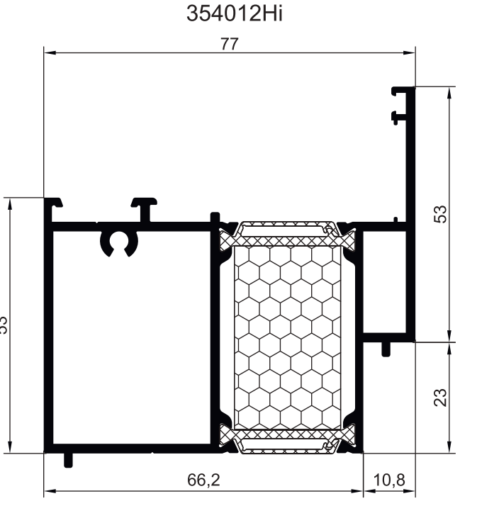
ПРОФИЛЬ ПОДСТАВКИ ПОД ЗАПОЛНЕНИЕ
