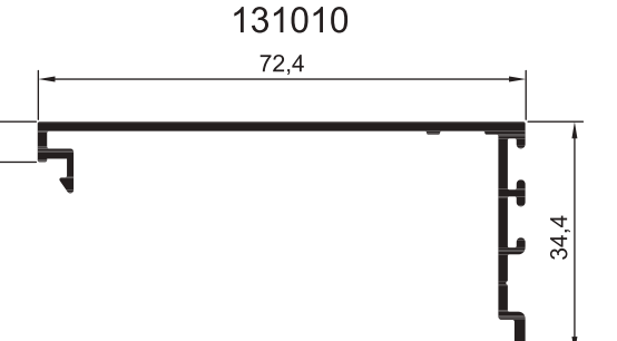
ПРОФИЛЬ КРЫШКИ ИМПОСТА
