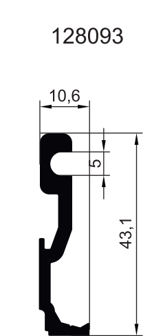
ПРОФИЛИ Т - ОБРАЗНОГО СОЕДИНЕНИЯ
