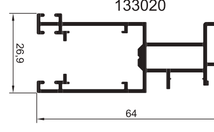
ПРОФИЛЬ ИМПОСТА АНТИМОСКИТНОЙ СЕТКИ
