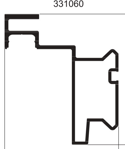
ПРОФИЛЬ УСИЛИТЕЛЯ ВНУТРЕННИЙ
