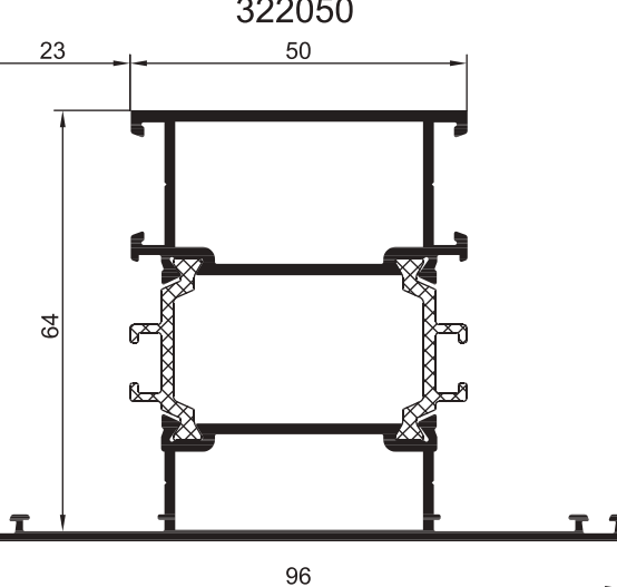
ПРОФИЛЬ КРЫШКИ СТОВРОКИ
