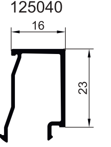
ПРОФИЛЬ ДВЕРНОЙ ШТУЛЬПОВЫЙ - ОТКРЫВАНИЕ ВНУТРЬ
