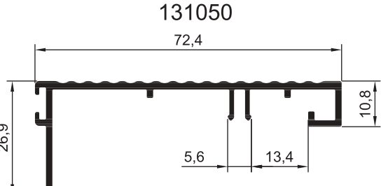
ПРОФИЛЬ ВНУТРЕННЕГО ПОРОГА
