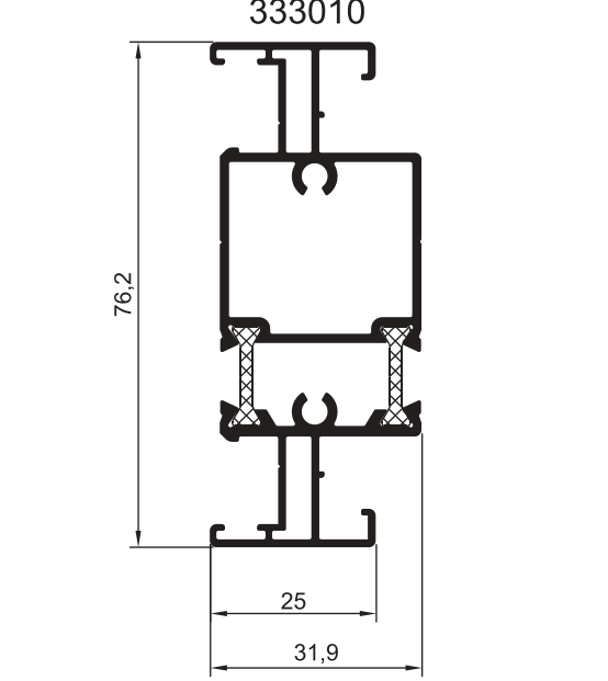
ПРОФИЛЬ ИМПОСТНЫЙ
