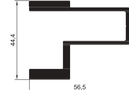
ПРОФИЛЬ УСИЛИТЕЛЯ НАРУЖНЫЙ
