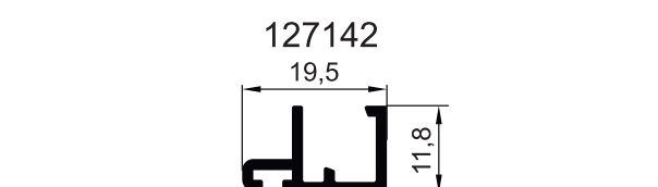
ПРОФИЛЬ ДВЕРНОГО ПРИТВОРА
