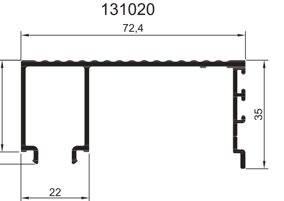
ПРОФИЛЬ КРЫШКИ РАМЫ
