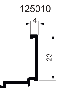
ПРОФИЛИ ШТАПИКА
