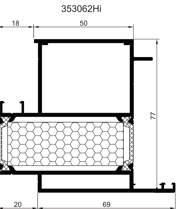
ДВЕРНОЙ РАМНОЙ ПРОФИЛЬ В ФАСАД - ОТКРЫВАНИЕ ВНУТРЬ
