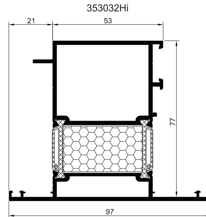
ПРОФИЛЬ ДВЕРНОЙ СТОВРОЧНЫЙ Z - ОБРАЗНЫЙ ПРОФИЛЬ
