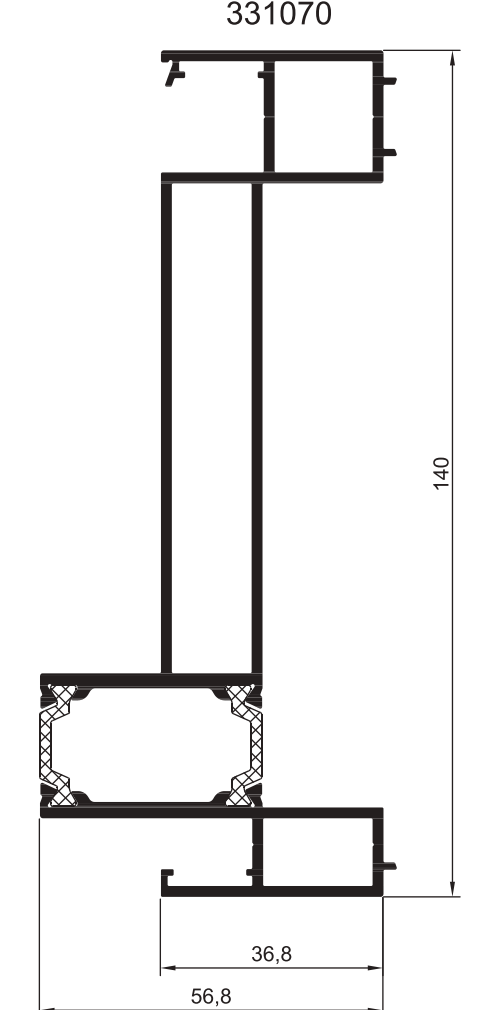
ПРОФИЛЬ АДАПТЕРА ДЛЯ УСТАНОВКИ В ФАСАД
