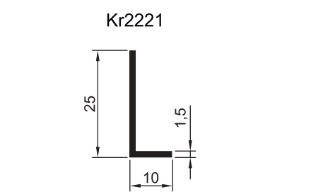
УГОЛОК
