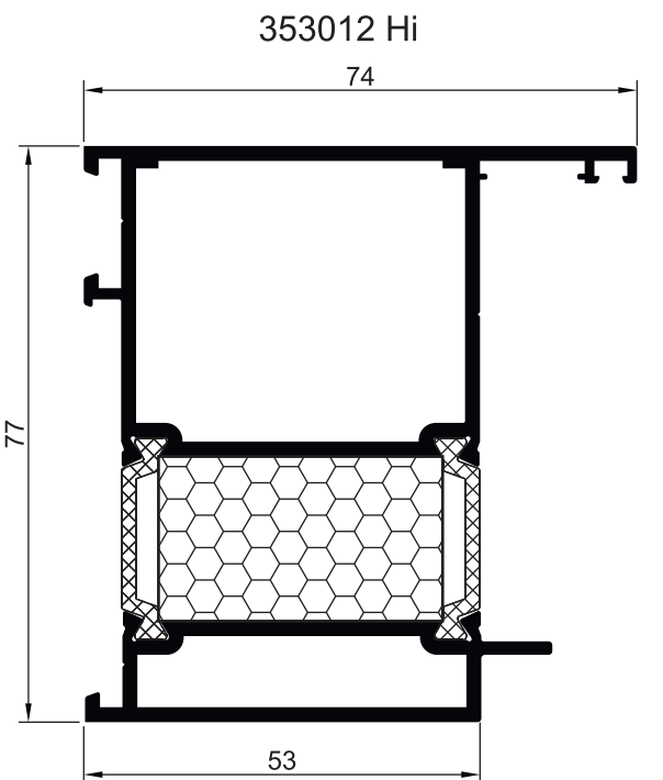
ПРОФИЛЬ ДВЕРНОЙ РАМНОЙ - ОТКРЫВАНИЕ ВНУТРЬ
