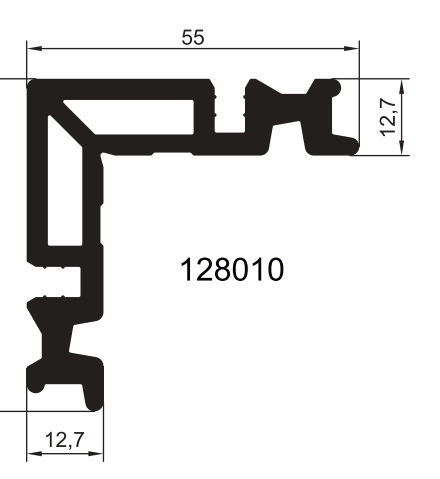
ПРОФИЛИ УГЛОВОГО СОЕДИНИТЕЛЯ
