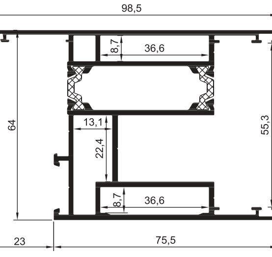
ПРОФИЛЬ СТЫКОВОЧНЫЙ
