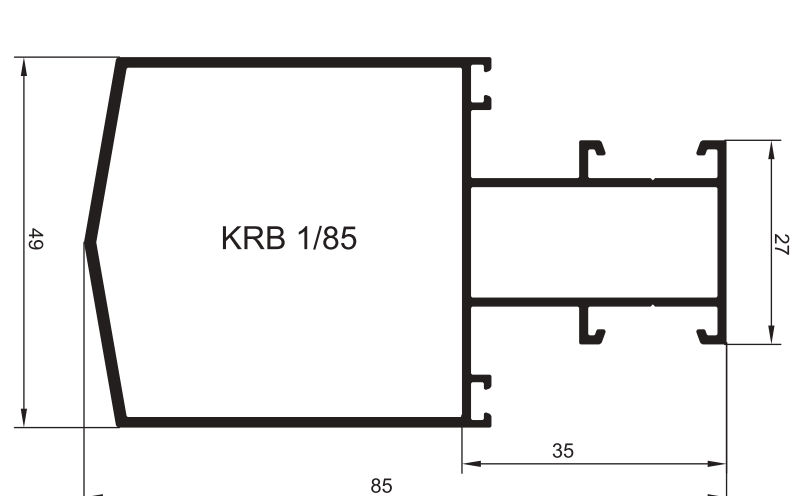
ПРОФИЛИ СТОЙКИ С НАРУЖНЫМ ПИЛОНОМ
