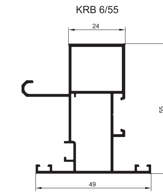
ПРОФИЛИ ОДНОРЕЗЬСОВОГО РИГЕЛЯ
