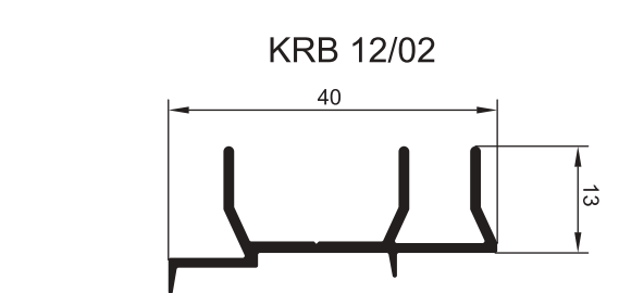
ПРОФИЛЬ ИМПОСТА ВЕРТИКАЛЬНОГО
