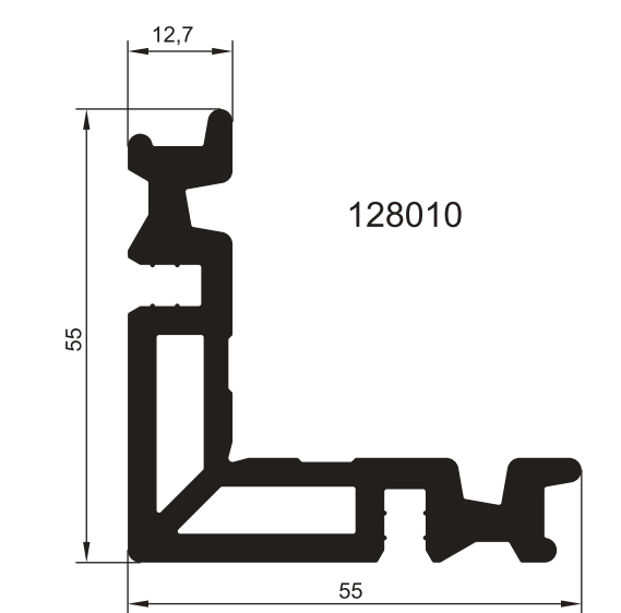
ПРОФИЛИ УГЛОВОГО СОЕДИНИТЕЛЯ
