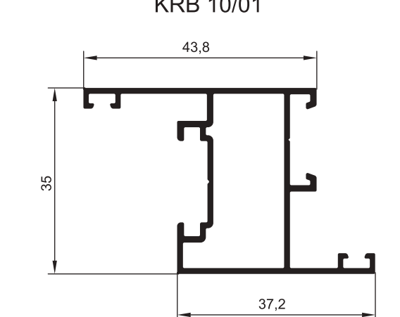
ПРОФИЛИ СТОЙКИ
