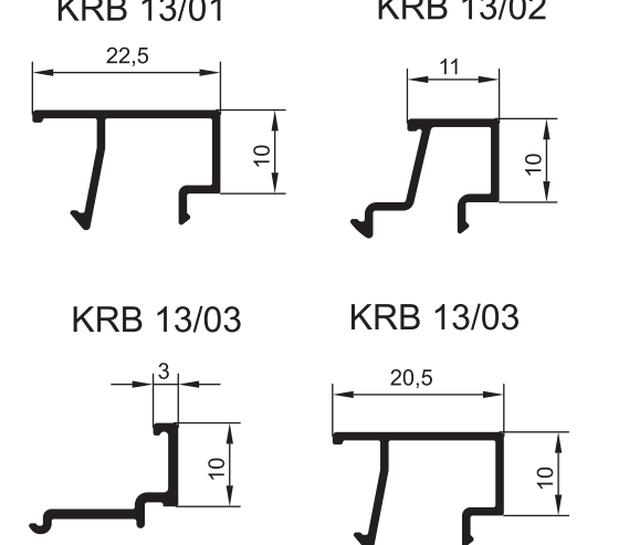
ПРОФИЛЬ ЗАКЛАДНОЙ СУХАРИ ИМПОСТА
