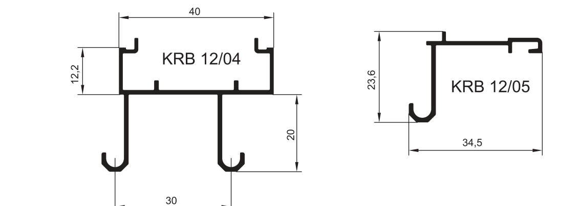
ПРОФИЛИ ЗАКЛАДНОЙ СУХАРИ СТОЙКИ
