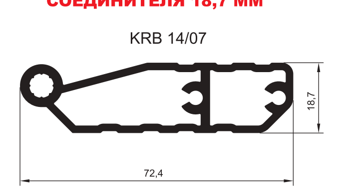
ПРОФИЛЬ УСИЛИТЕЛЯ СТОЙКИ С УЗКИМ ВНУТРЕННИМ ПИЛОНОМ
