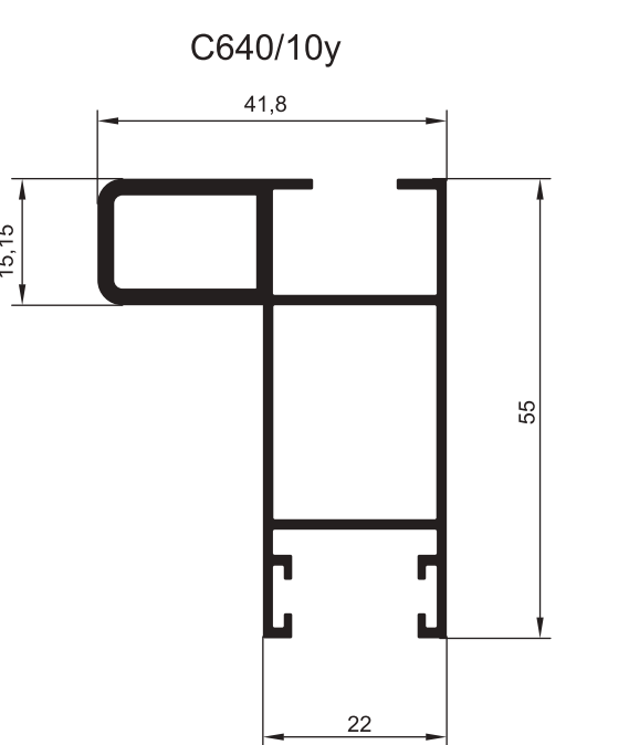
ПРОФИЛИ СТОЙКИ ЦЕНТРАЛЬНОЙ УСИЛЕННОЙ
