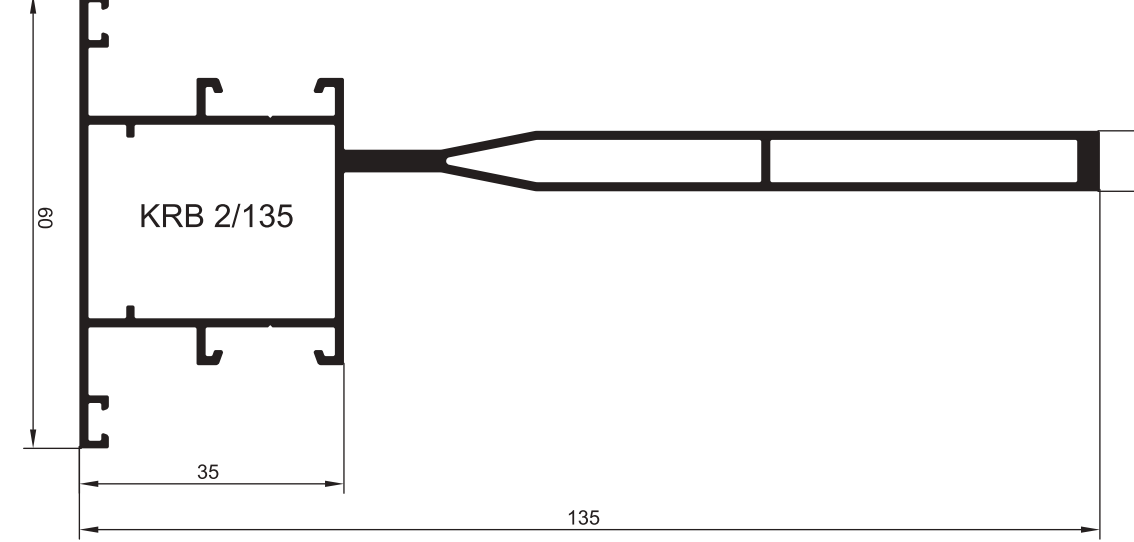
ПРОФИЛИ СТОЙКИ С УЗКИМ ВНУТРЕННИМ ПИЛОНОМ
