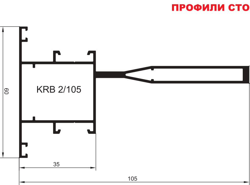
ПРОФИЛИ СТОЙКИ С УЗКИМ ВНУТРЕННИМ ПИЛОНОМ
