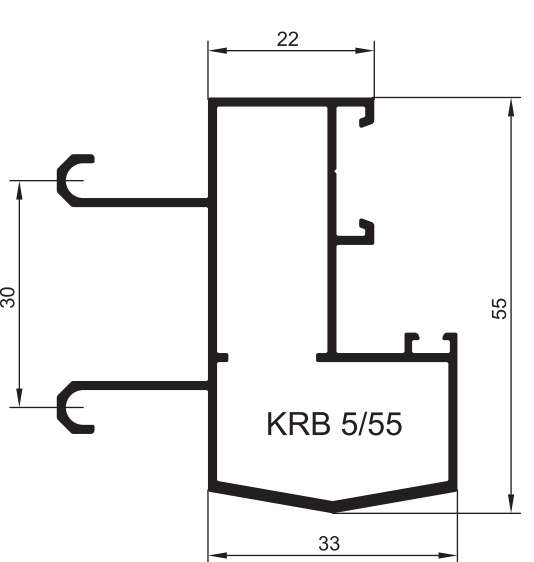
ПРОФИЛИ РИГЕЛЯ
