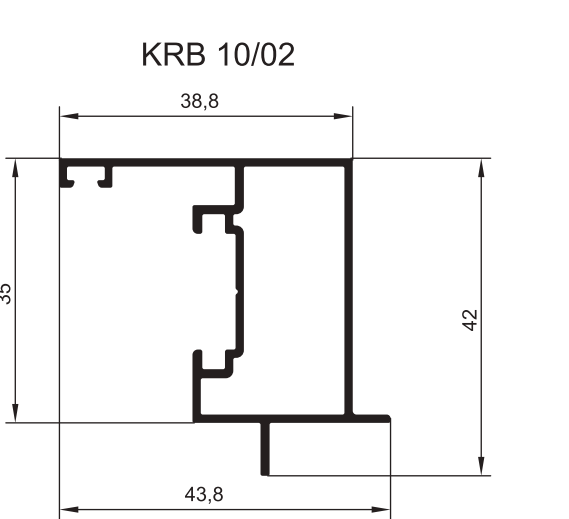
ПРОФИЛИ СТОЙКИ СТРУКТУРНОЙ
