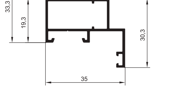
ПРОФИЛИ РИГЕЛЯ РАЗРЫВА
