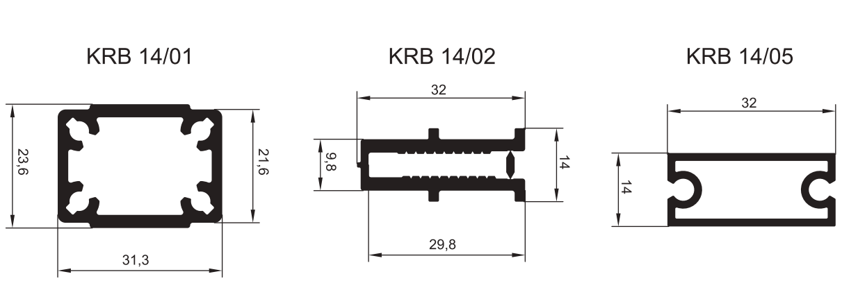
ПРОФИЛЬ РАМЫ 35 ММ
