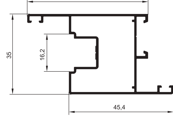
ПРОФИЛИ РИГЕЛЯ РАЗРЫВА
