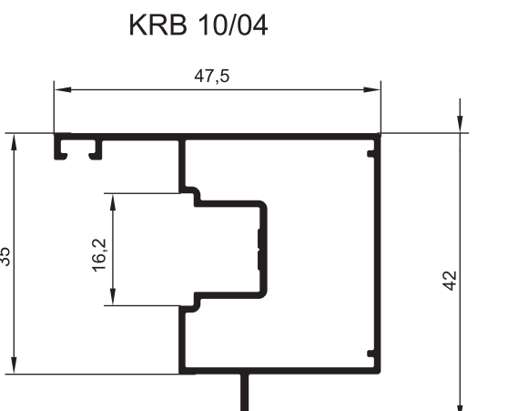
ПРОФИЛИ СТОЙКИ БОКОВОЙ УСИЛЕННОЙ
