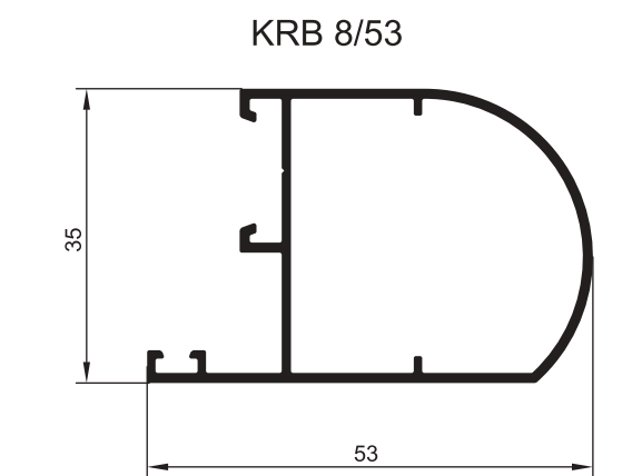
ПРОФИЛЬ ОГРАНИЧИТЕЛЯ СТВОРОК
