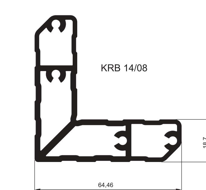
ПРОФИЛЬ УГЛОВОГО ШАРНИРНОГО СОЕДИНИТЕЛЯ 18,7 ММ
