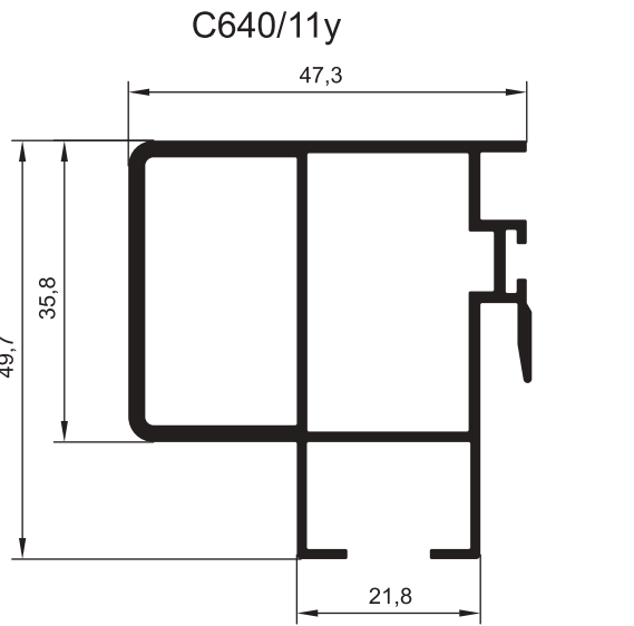
ПРОФИЛИ ШТАПИКОВ
