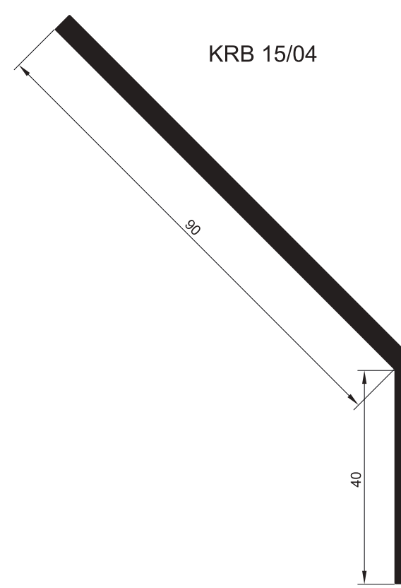
ПРОФИЛЬ УГЛОВОЙ ШИНЫ
