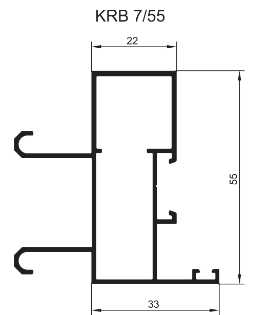
ПРОФИЛИ ДВУХРЕЗЬСОВОГО РИГЕЛЯ
