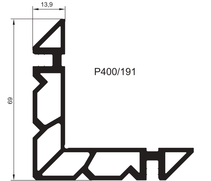
ПРОФИЛИ СТОЙКИ БОКОВОЙ УСИЛЕННОЙ
