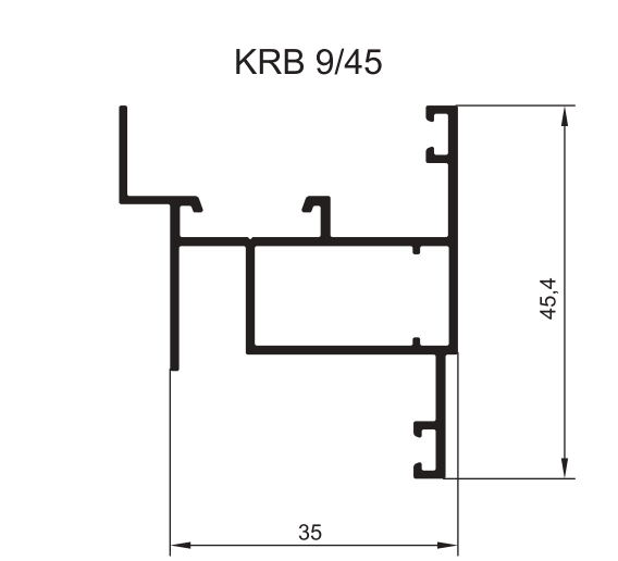
ПРОФИЛИ РИГЕЛЯ РАЗРЫВА
