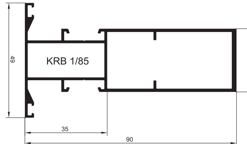
ПРОФИЛИ СТОЙКИ С ШИРОКИМ ВНУТРЕННИМ ПИЛОНОМ
