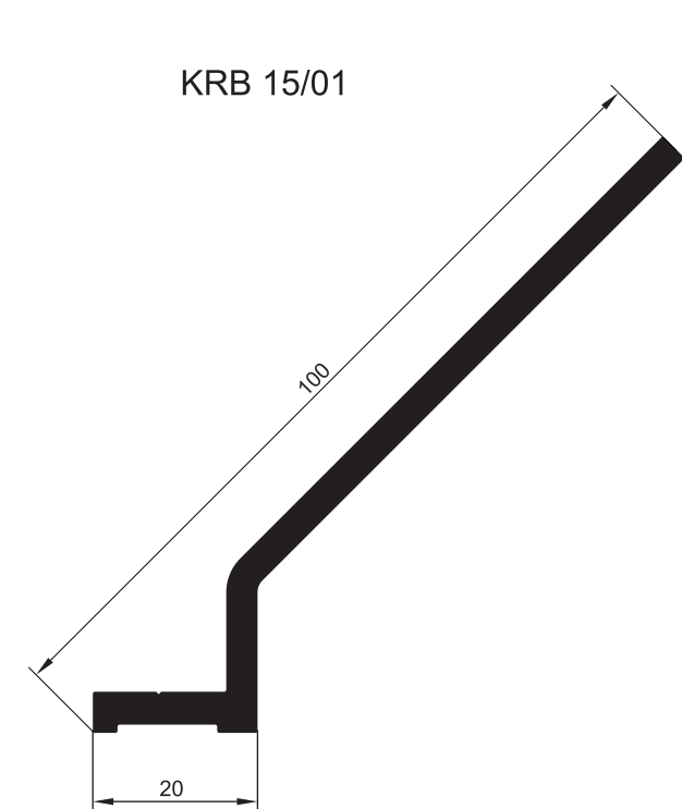
ПРОФИЛЬ УСИЛИТЕЛЯ СТОЙКИ С УЗКИМ ВНУТРЕННИМ ПИЛОНОМ
