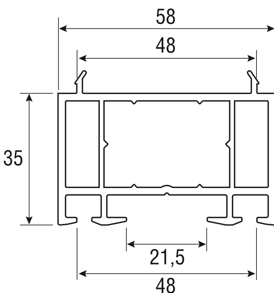
2.1.18 Статический усилитель арт. 5871
