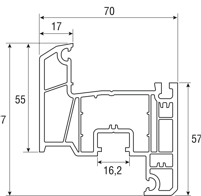
4.2.3 Профиль створки дверной внутреннего открывания арт. 5815
