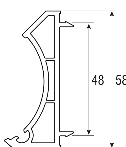
2.1.11 Профиль адаптер к трубе для эркерных окон арт. 5813
