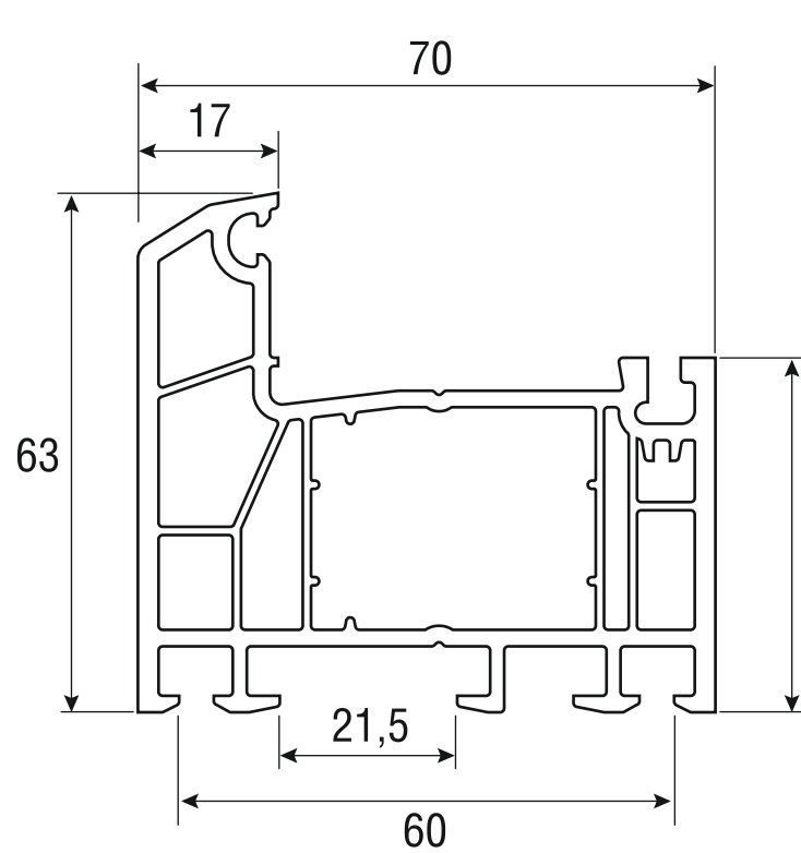
4.2.2 Профиль створки дверной/импоста наружного открывания арт. 5805
