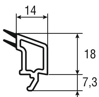
2.1.9 Профиль соединительный арт. 5810
