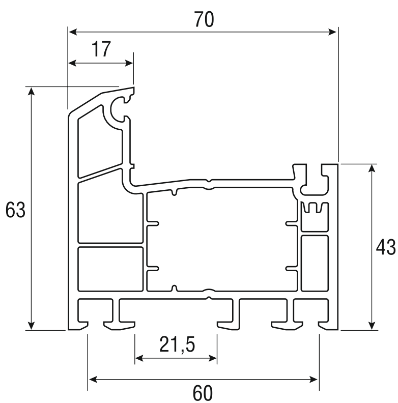
3.1.5 Профиль створки арт. 7502
