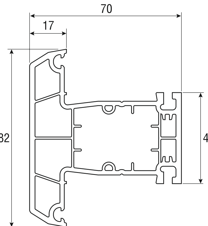
4.2.1 Профиль рамы дверной арт. 5804
