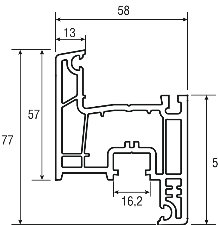
3.1.3 Профиль импоста арт. 7303
