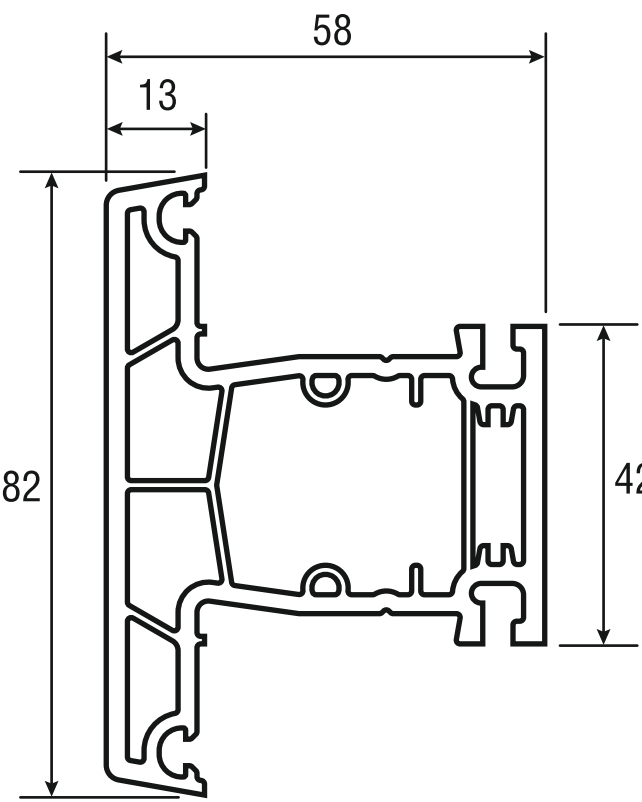
3.1.4 Профиль рамы арт. 7501
