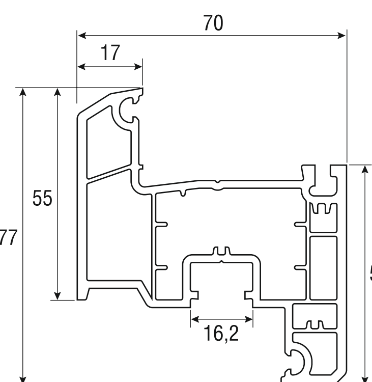
3.1.6 Профиль импоста арт. 7503
