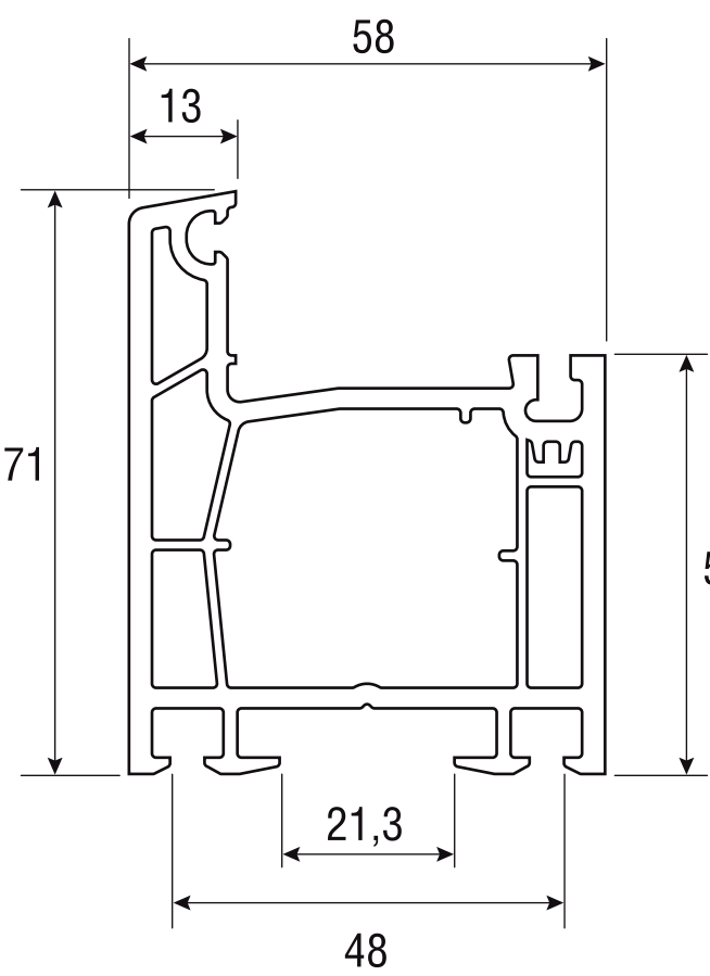
4.2.1 Профиль рамы дверной арт. 5804
