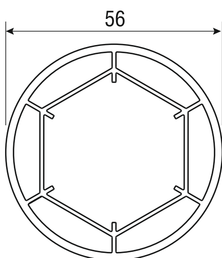
3.1.11 Профиль соединительный арт. 7010
