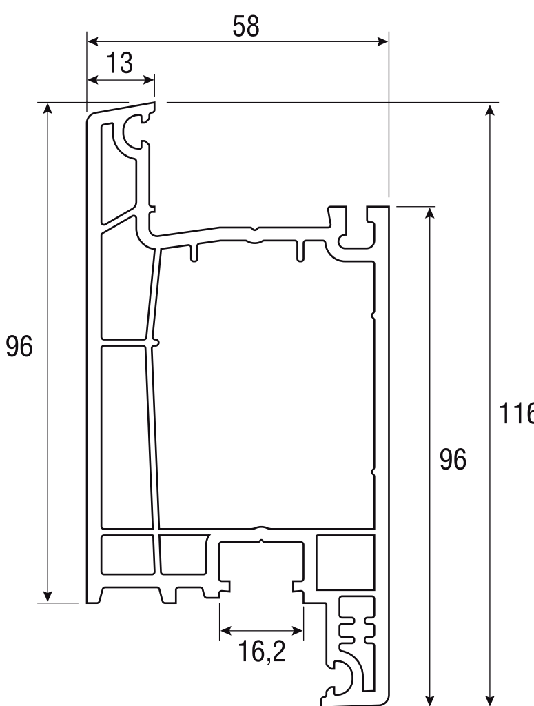
4.2.3 Профиль створки дверной внутреннего открывания арт. 5815
