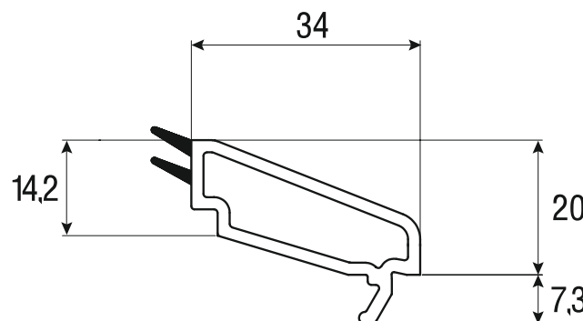
2.1.11 Профиль адаптер к трубе для эркерных окон арт. 5813
