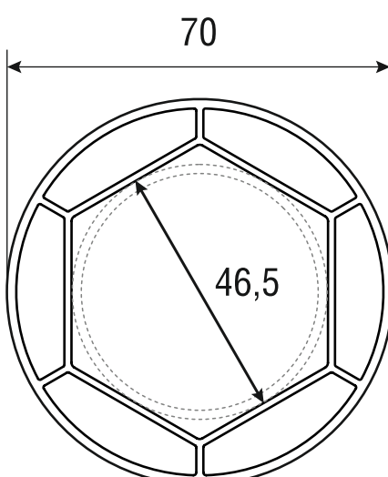
3.1.15 Труба ПВХ для эркерных окон арт. 7013
