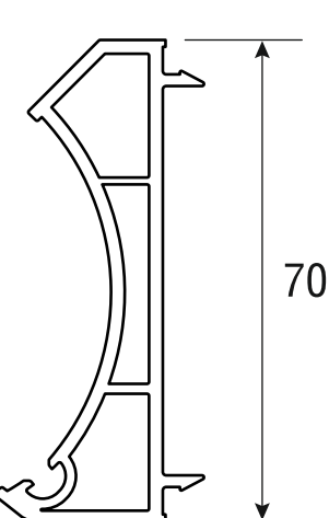
3.1.14 Адаптер к трубе для эркерных окон арт. 7014
