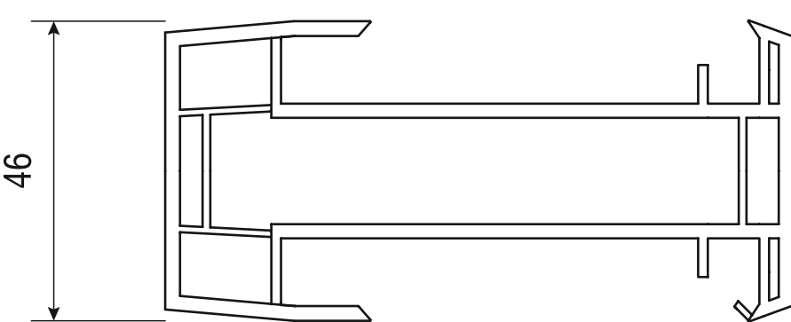
3.1.14 Адаптер к трубе для эркерных окон арт. 7014
