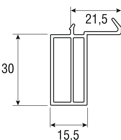
2.1.12 Профиль штульпа арт. 5806
