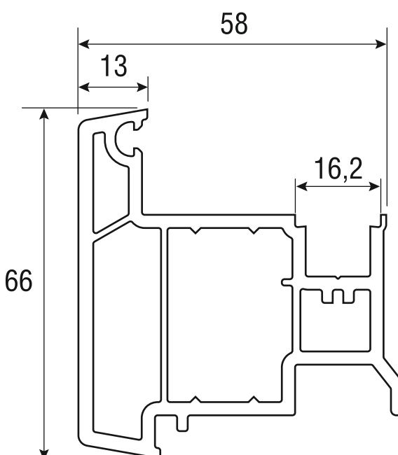
2.1.12 Профиль штульпа арт. 5806
