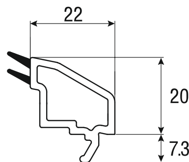
3.1.8 Профиль штапика 22 мм с коэкструдированным уплотнением арт.7524
