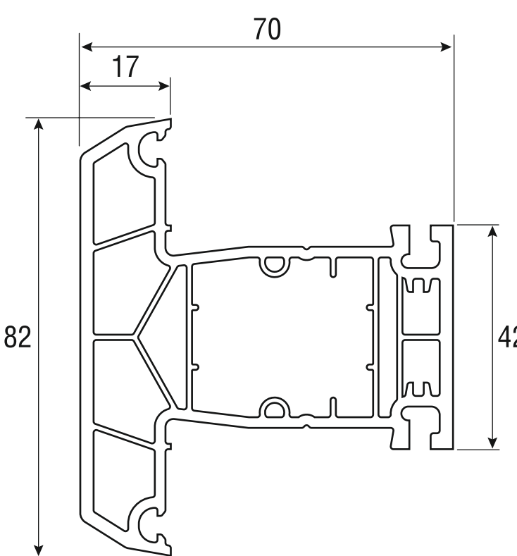
3.1.6 Профиль импоста арт. 7503
