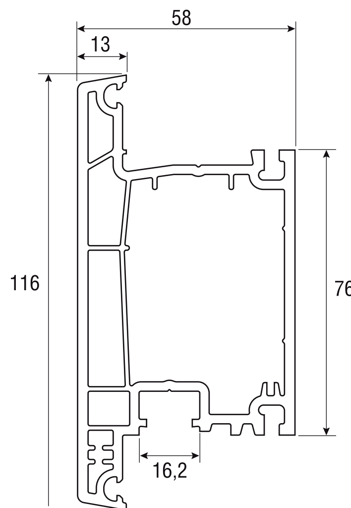
4.2.2 Профиль створки дверной/импоста наружного открывания арт. 5805
