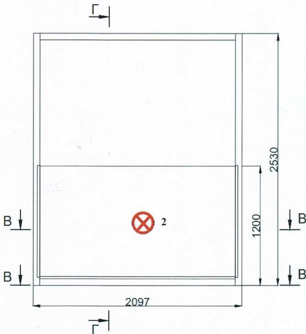
Рис 4. Схема приложения ударной испытательной нагрузки к ограждающему экрану конструкции (2- центр экрана заполнения ограждения)
