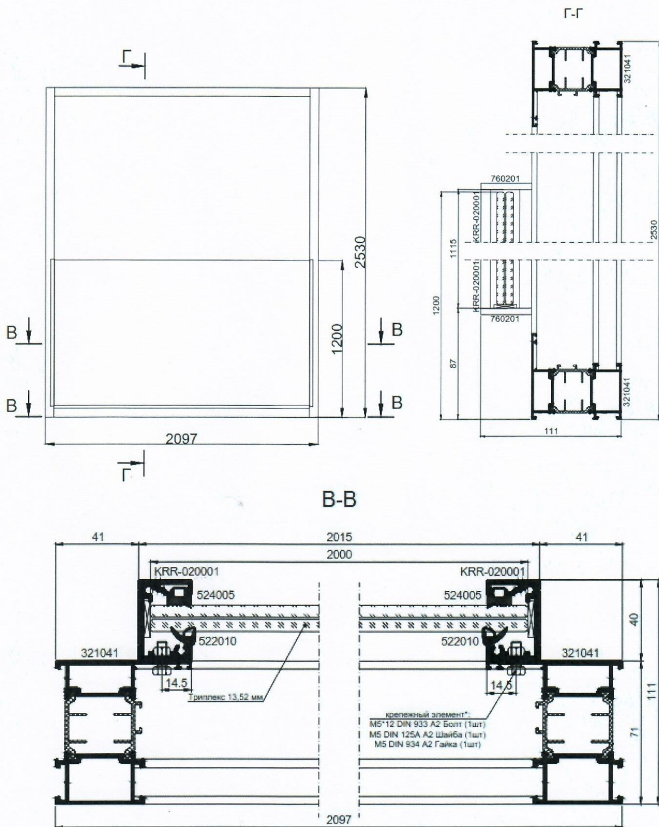
Рис 2. Фрагмент светопрозрачной ограждающей конструкции системы французских балконов «KRAUSS KRR», регистрационный номер ИЛ 4958-25.
