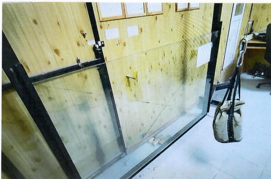
Фото 8. Общий вид после удара (точка 2), высота падения 1200мм. Образец не имеет видимых разрушений. Целостность образца не нарушена, остекление не выпало.
