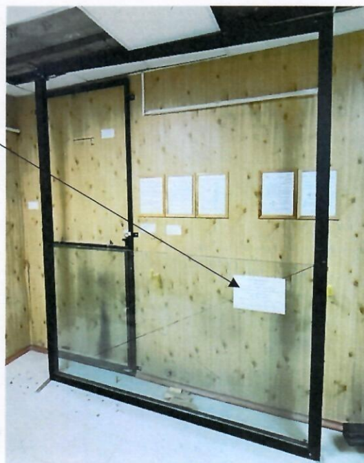
Фото 3, 4. Образец рег. № 4958-25. При воздействии нагрузки конструкция не имеет видимых деформаций, остаточная деформация отсутствует, ограждающий экран не выпал.
