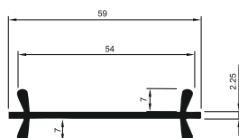
Профиль соединительный Арт. 6010
