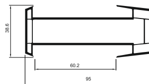
Профиль соединительный усиливающий Арт. 6019
