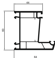
Профиль рамы Арт. 6001
