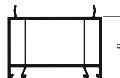
Профиль расширительный 40 мм. Арт. 6012
