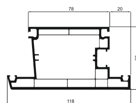
Профиль створки дверной Арт. 6005
