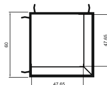
Профиль соединительный угловой Арт. 6090
