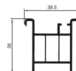
Профиль подставочный Арт. 6009
