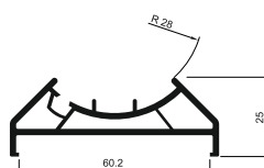
Профиль адаптера к трубе Арт. 6013
