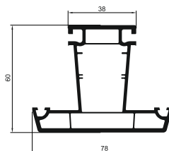
Профиль импоста Арт. 6003
