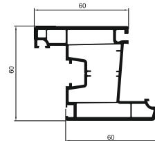
Профиль створки Арт. 6002
