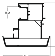
Профиль штапика Арт. 6006
